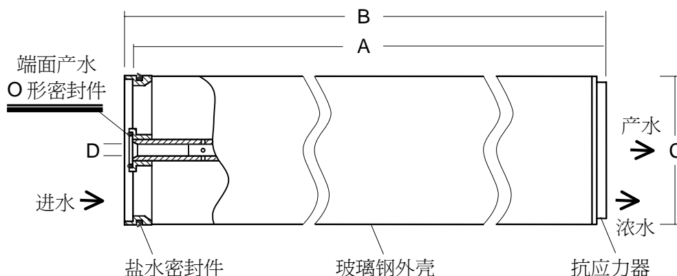
外形尺寸 - 英寸 (mm)
